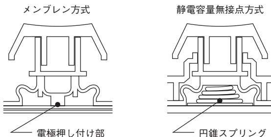
●図-1 メンブレン方式と静電容量無接点方式●
